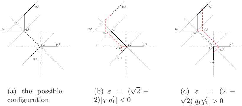
Fig. 3. Proof of Lemma 8.
